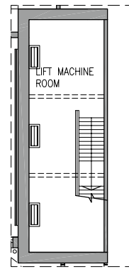
PART PLAN AT 22/F 二十二樓部分平面圖
