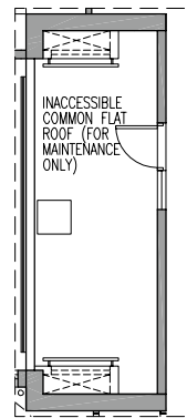
PART PLAN AT 25/F 二十五樓部分平面圖
