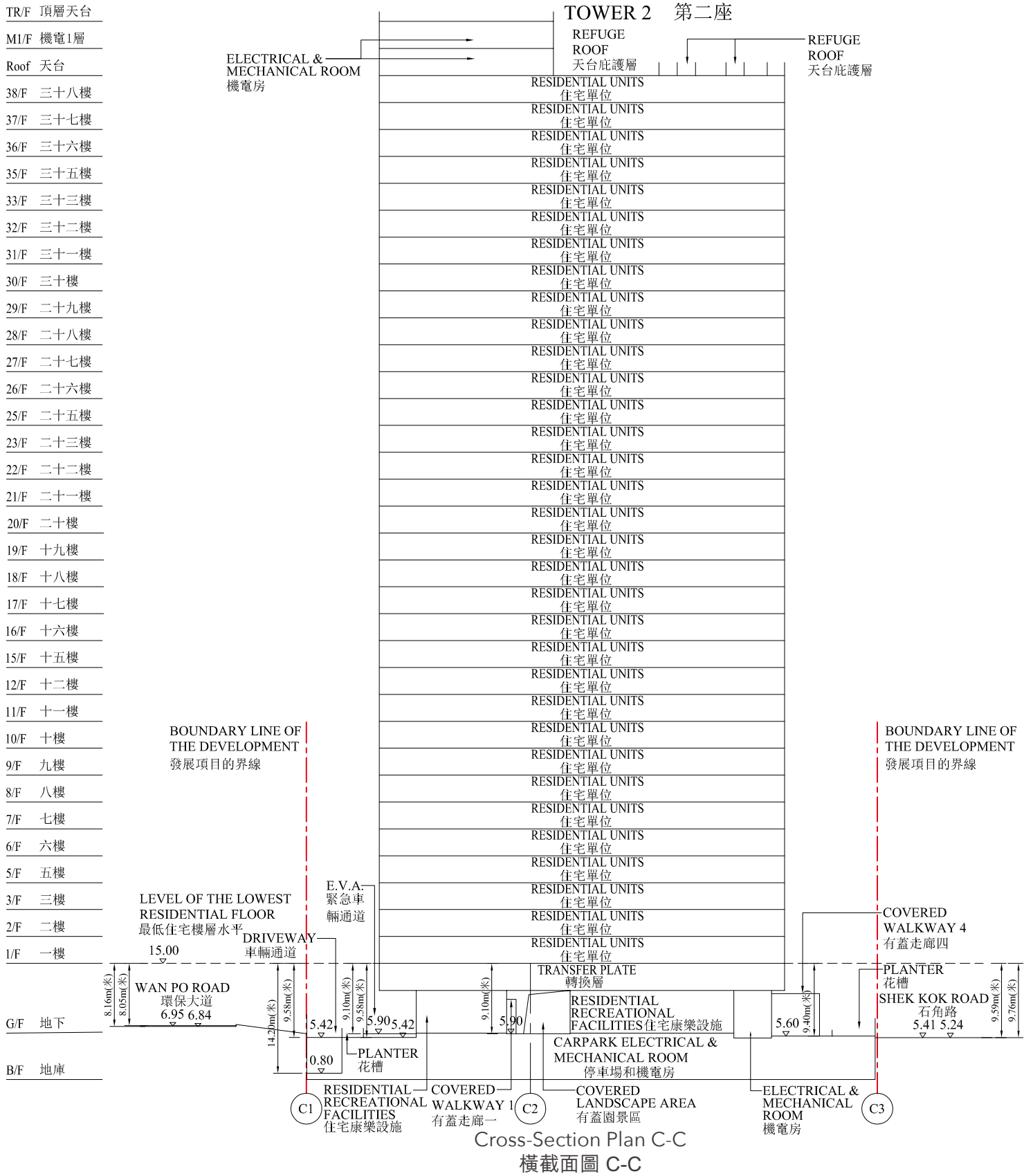
Cross-Section Plan C-C 橫截面圖 C-C
